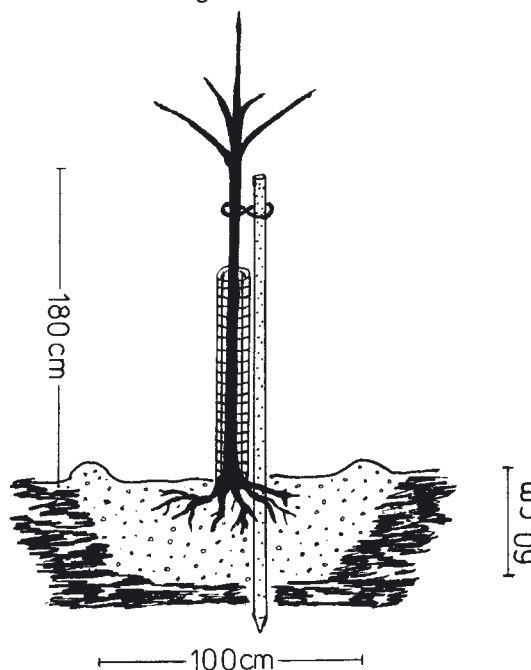
Fachgerecht gepflanzter Obstbaum Zeichnung: Thomas Grunwald
